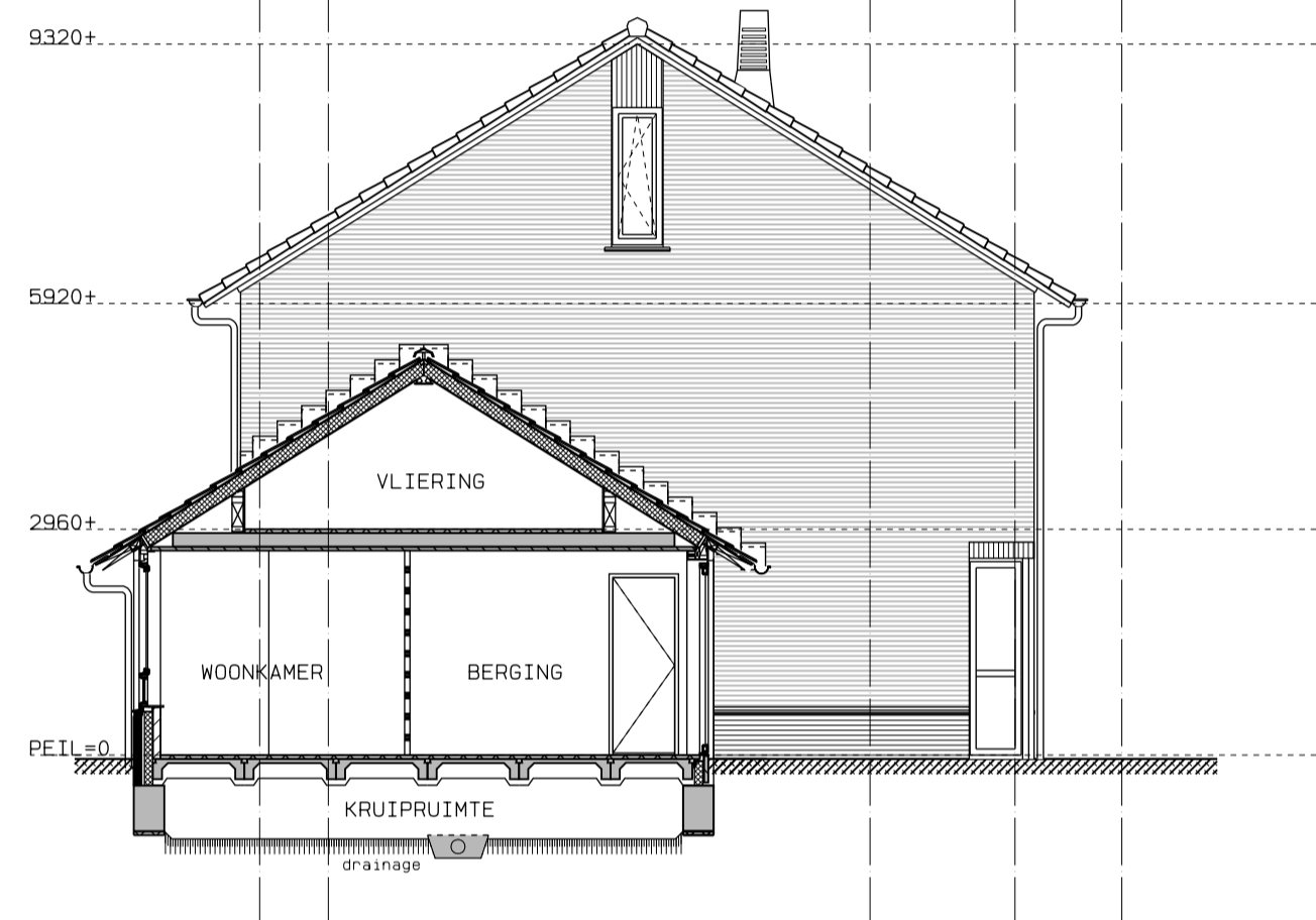
doorsnede B-B BOUWNR. 142
