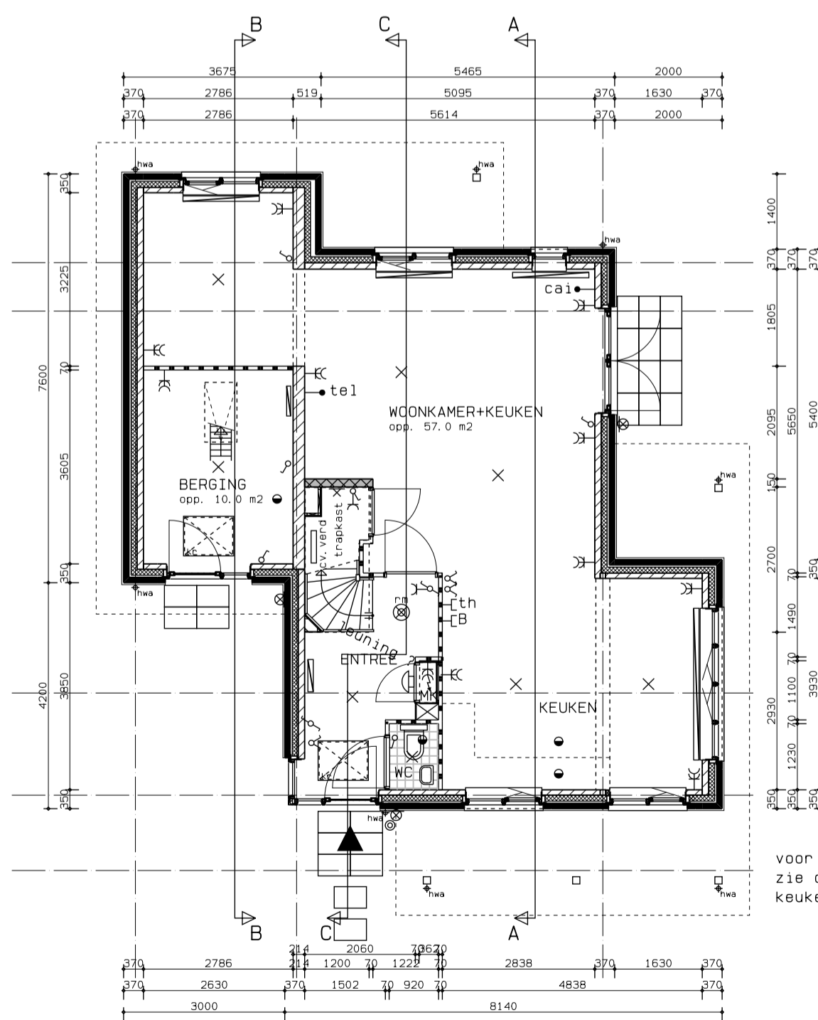
begane Grond BOUWNR. 142
