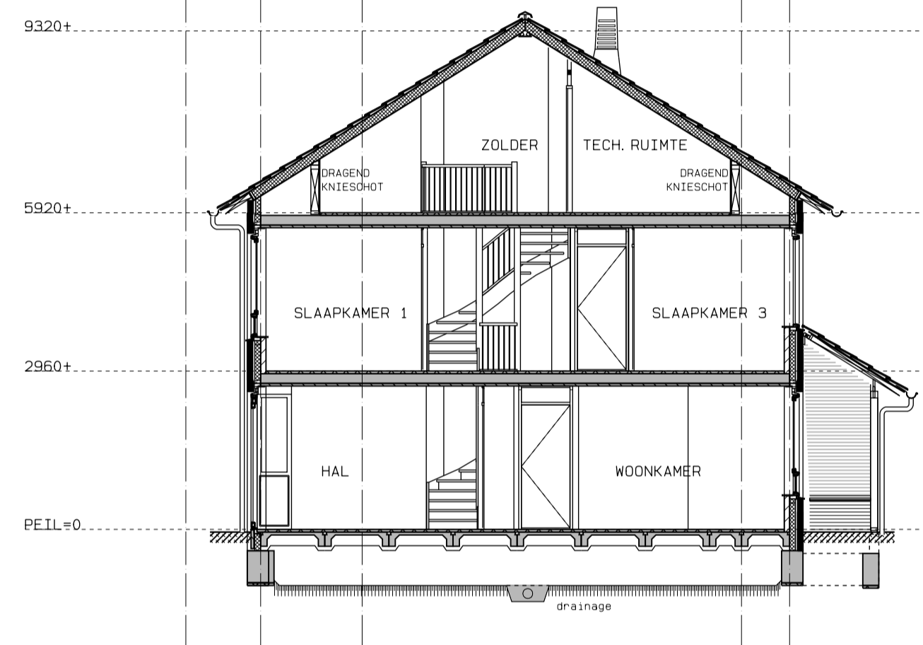
doorsnede C-C BOUWNR. 142
