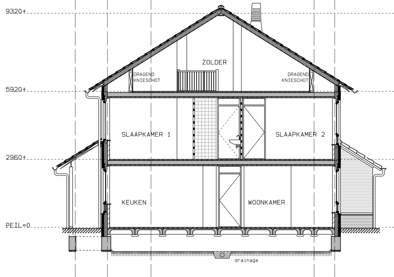
doorsnede A-A BOUWNR. 142
