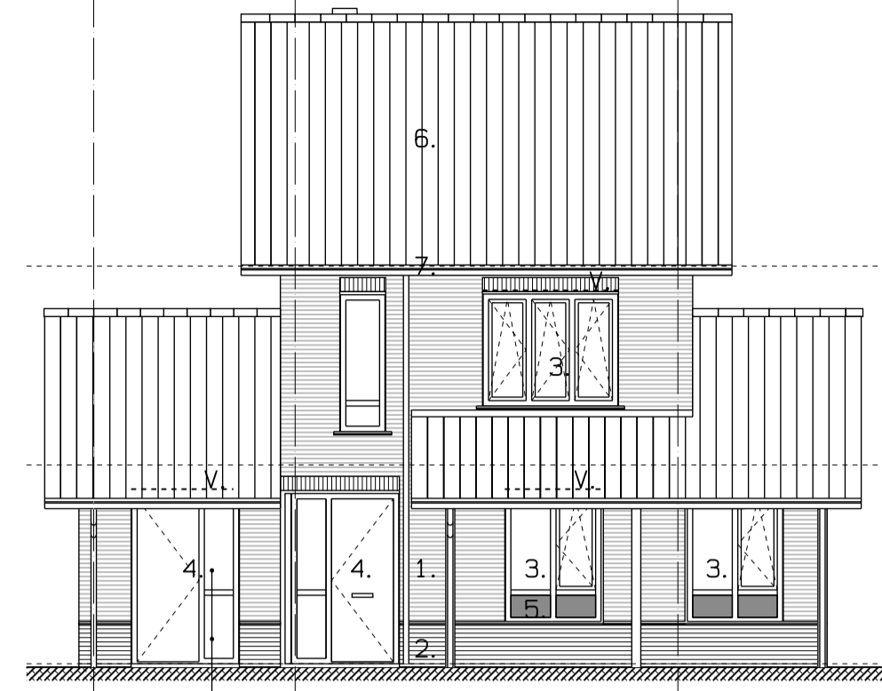
voorgevel BOUWNR. 142
