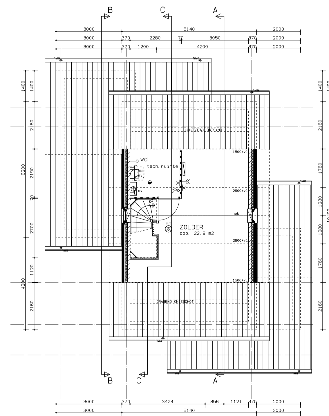
2e verdieping BOUWNR. 142
