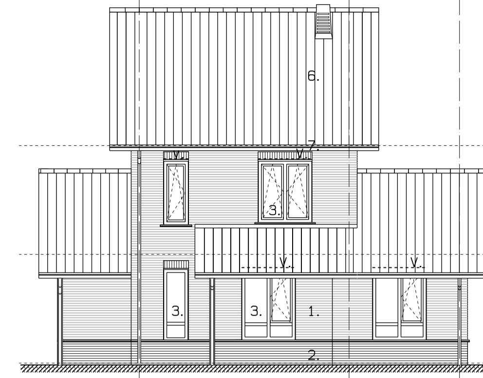
achtergevel BOUWNR. 142
