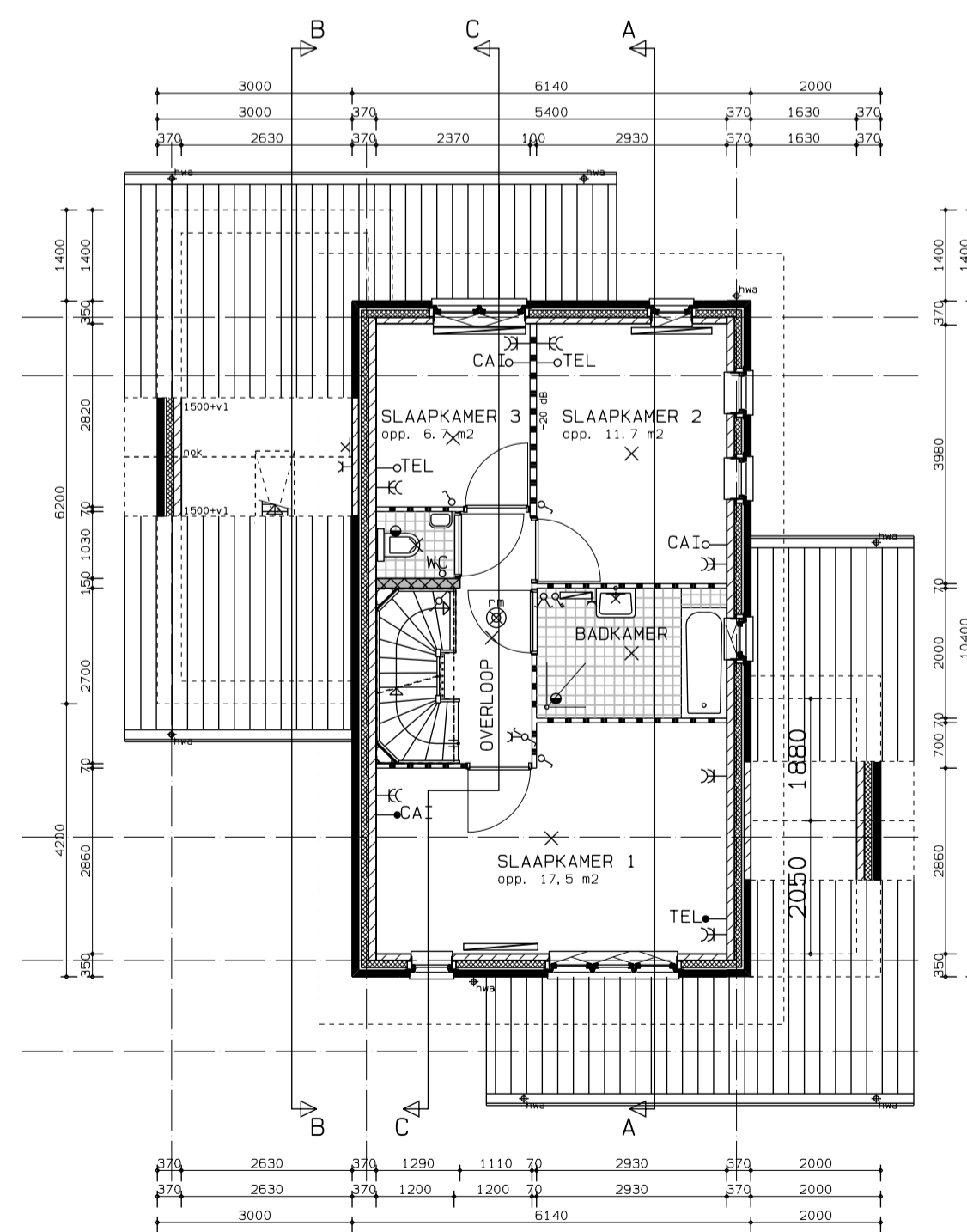
1e verdieping BOUWNR. 142
