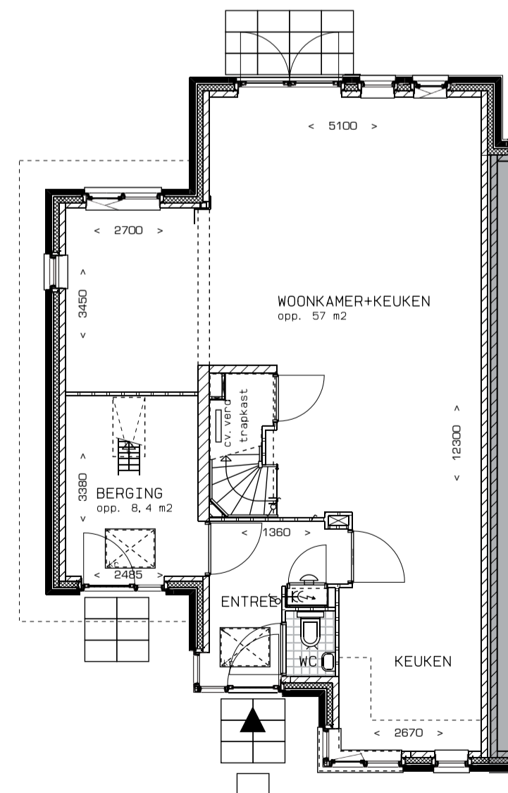
Begane grond • uitbouw 1200 mm achtergevel • schacht voor wtw douche bouwnummers: 2, 6, 7, 10, 150 en 154 bouwnummers gespiegeld: 1, 3, 8, 9, 153 en 157 schaal 1:100
