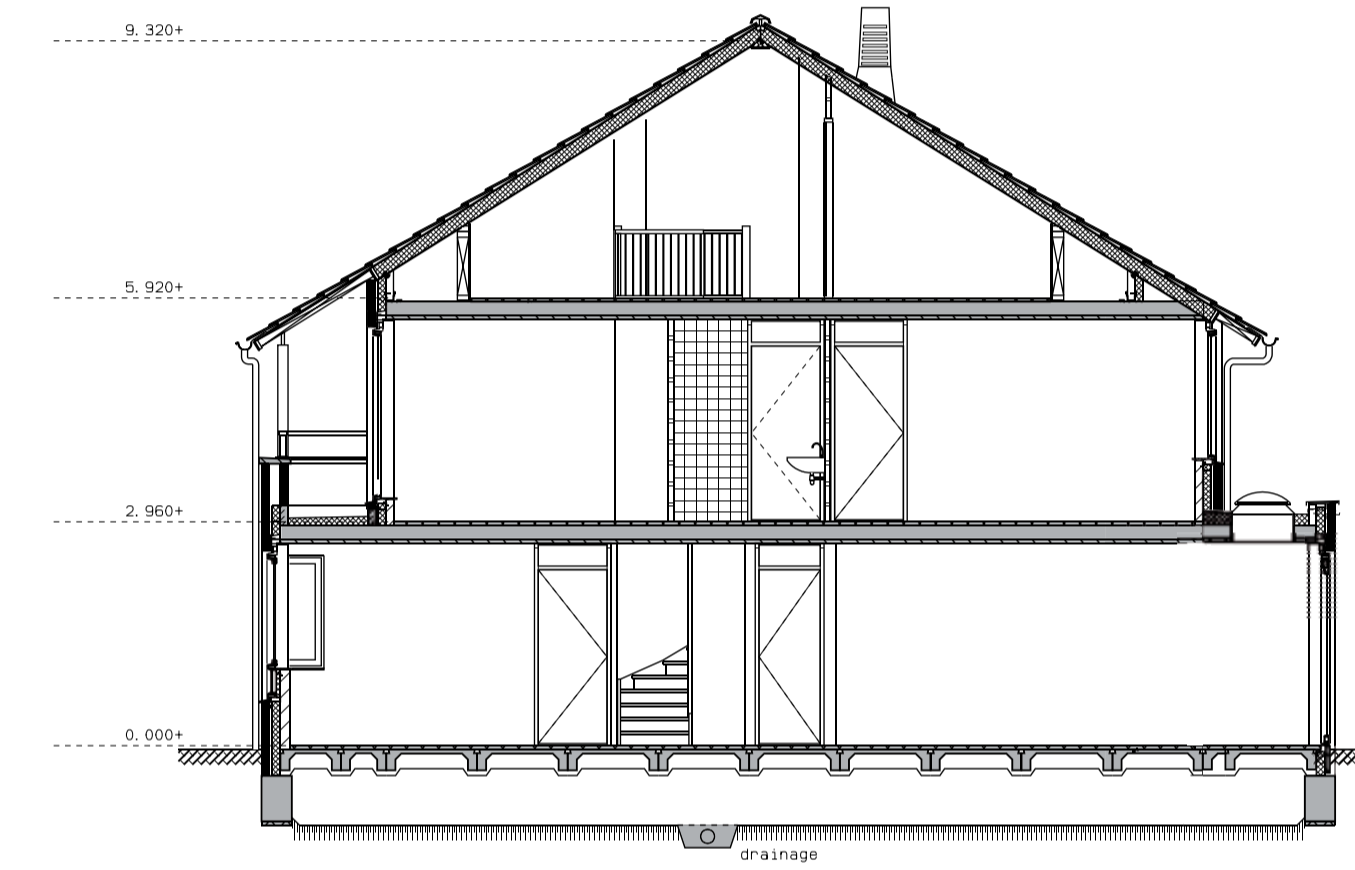
Doorsnede • uitbouw 2400 mm + lichtkoepel i.c.m. uitbouw 900 mm 1e verdieping bouwnummers: 2, 6, 7, 10, 150 en 154 bouwnummers gespiegeld: 1, 3, 8, 9, 153 en 157 schaal 1 : 100
