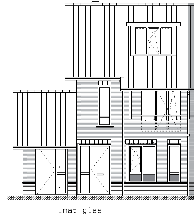
Voorgevel • aanzicht dakkapel voorgevel bouwnummers: 2, 6, 7, 10, 150 en 154 bouwnummers gespiegeld: 1, 3, 8, 9, 153 en 157 schaal 1:100
