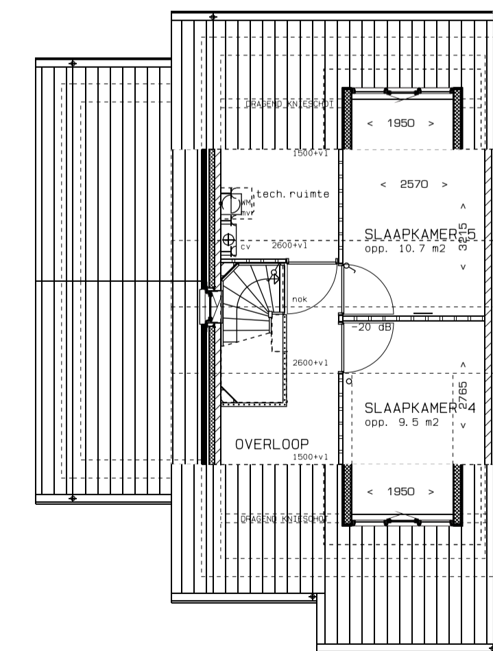
Tweede verdieping • dakkapel voor- en achtergevel bouwnummers: 2, 6, 7, 10, 150 en 154 bouwnummers gespiegeld: 1, 3, 8, 9, 153 en 157 schaal 1 : 100
