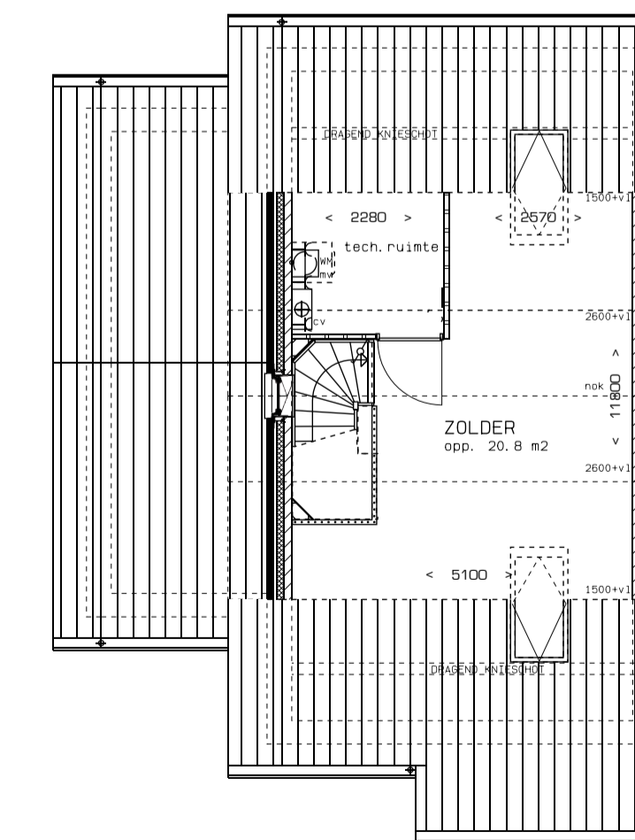
Tweede verdieping • dakraam voor- en achtergevel bouwnummers: 2, 6, 7, 10, 150 en 154 bouwnummers gespiegeld: 1, 3, 8, 9, 153 en 157 schaal 1 : 100
