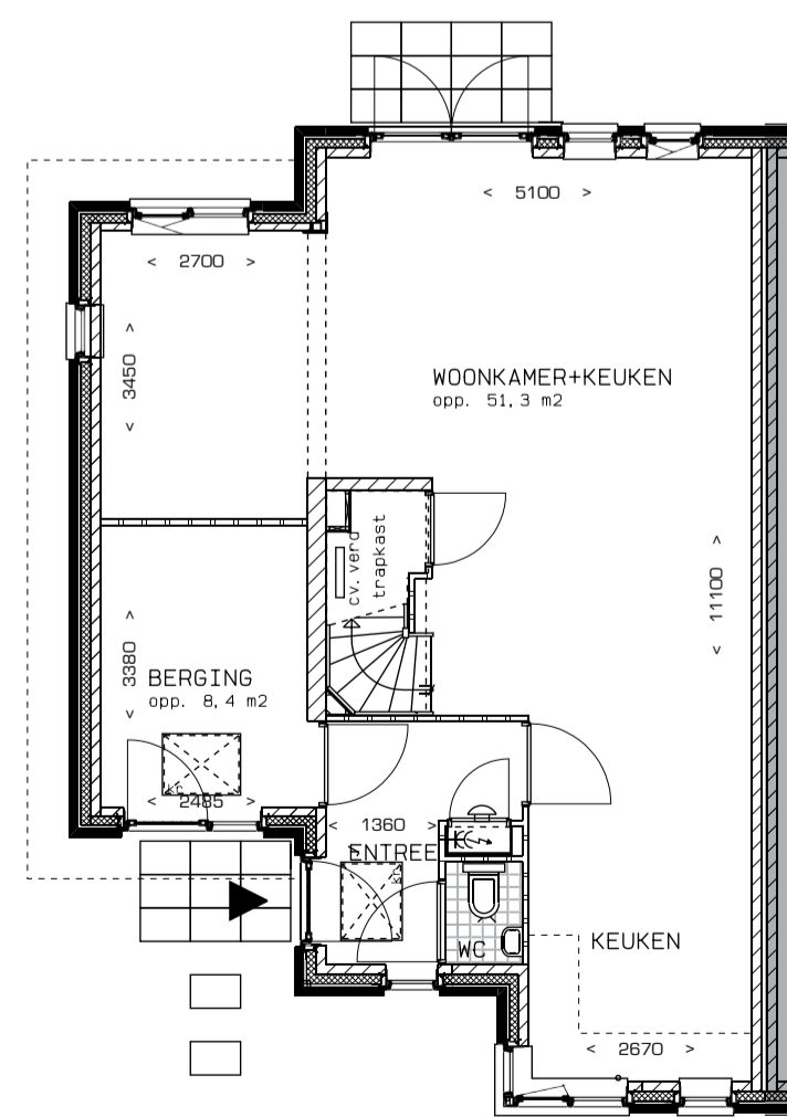
Begane grond • entree bij slaapkamer 6 bouwnummers: 2, 6, 7, 10, 150 en 154 bouwnummers gespiegeld: 1, 3, 8, 9, 153 en 157 schaal 1 : 100
