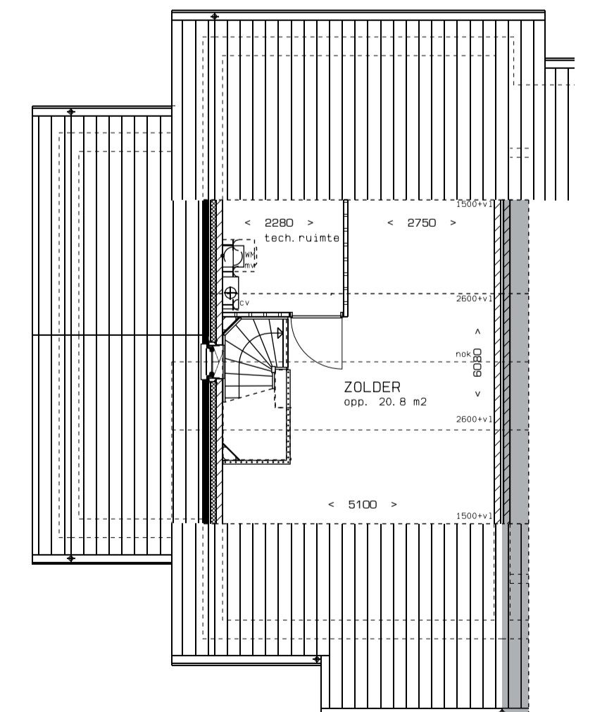
Tweede verdieping • uitbouw 900 mm bouwnummers: 150 en 154 schaal 1 : 100
