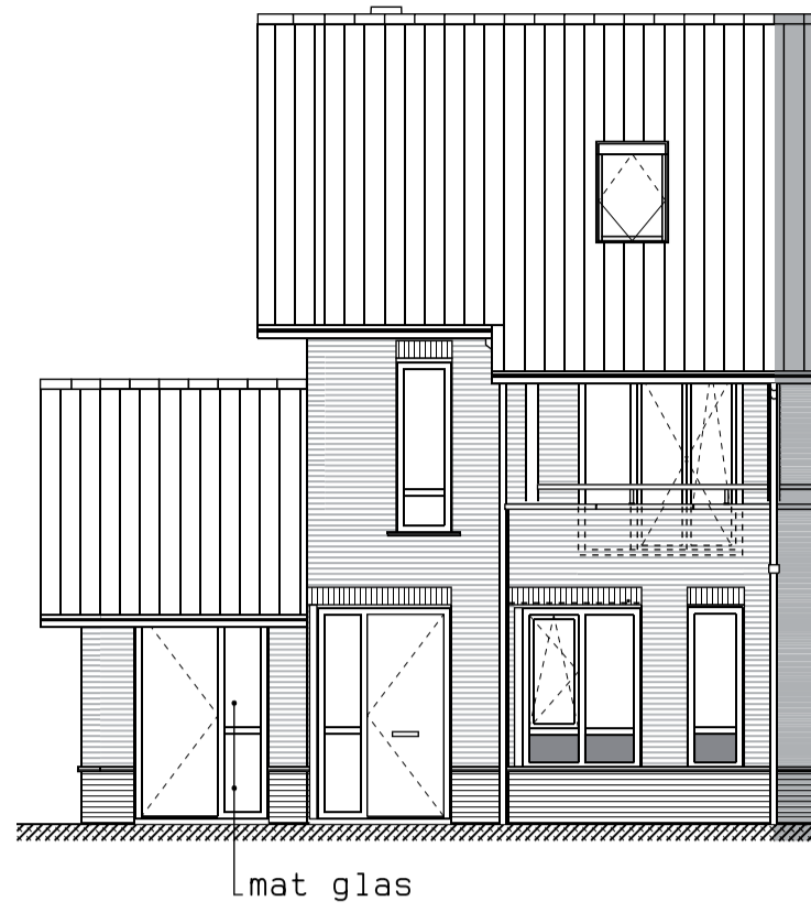
Voorgevel • aanzicht dakraam bouwnummers: 2, 6, 7, 10, 150 en 154 bouwnummers gespiegeld: 1, 3, 8, 9, 153 en 157 schaal 1:100
