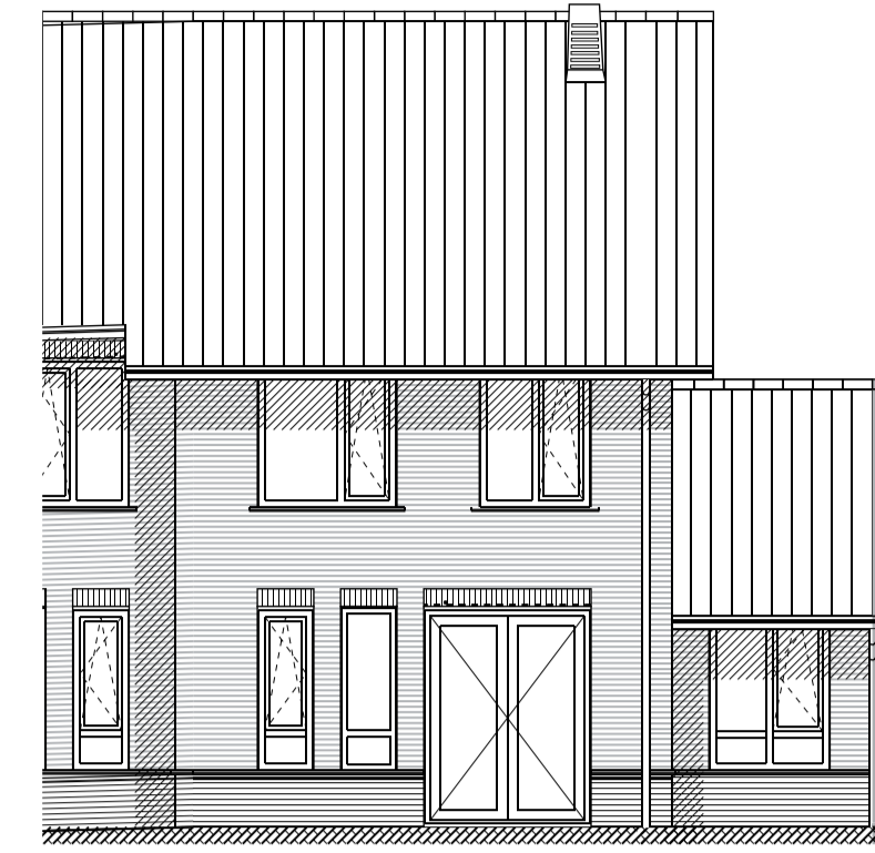
Achtergevel • aanzicht uitbouw 900 mm bouwnummers: 2, 6, 7, 10, 150 en 154 bouwnummers gespiegeld: 1, 3, 8, 9, 153 en 157 schaal 1 : 100
