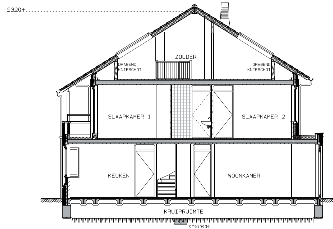
Doorsnede • doorsnede dakraam voor- en achtergevel • uitbouw 1200 mm bouwnummers: 2, 6, 7, 10, 150 en 154 bouwnummers gespiegeld: 1, 3, 8, 9, 153 en 157 schaal 1:100
