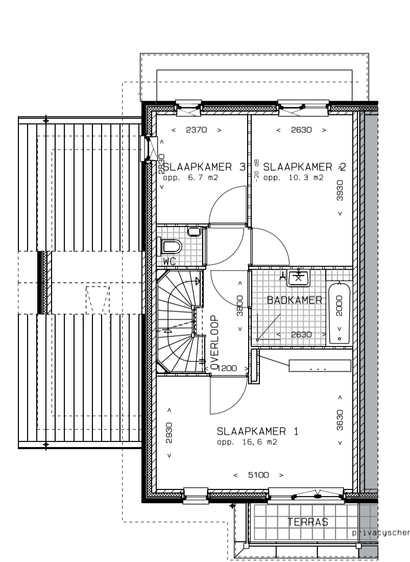
Eerste verdieping • dak uitbouw 1200 mm • schacht voor wtw douche bouwnummers: 2, 6, 7, 10, 150 en 154 bouwnummers gespiegeld: 1, 3, 8, 9, 153 en 157 schaal 1:100
