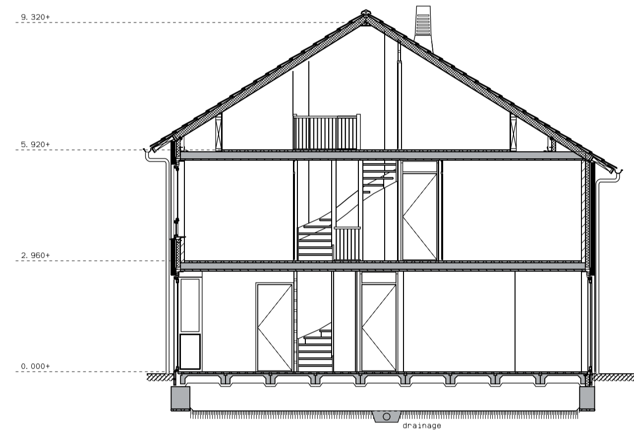
Doorsnede • uitbouw 900 mm bouwnummers: 2, 6, 7, 10, 150 en 154 bouwnummers gespiegeld: 1, 3, 8, 9, 153 en 157 schaal 1 : 100
