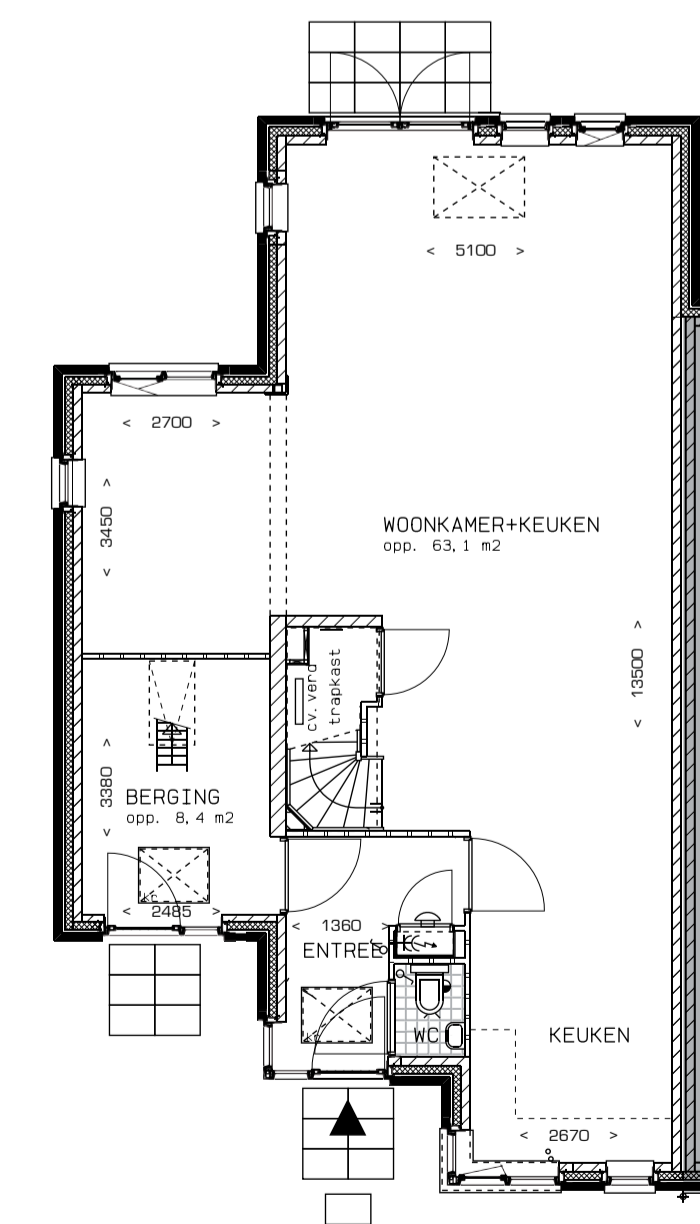
Begane grond • uitbouw 2400 mm achtergevel + lichtkoepel i.c.m. uitbouw 900 mm 1e verdieping • raam in zijgevel uitbouw 2400 mm bouwnummers: 2, 6, 7, 10, 150 en 154 bouwnummers gespiegeld: 1, 3, 8, 9, 153 en 157 schaal 1:100
