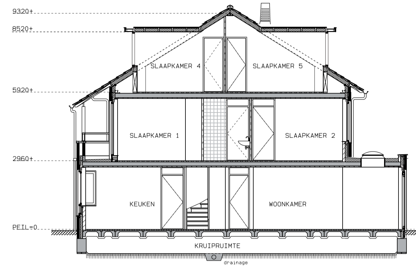
Doorsnede • doorsnede dakkapel voor- en achtergevel • uitbouw 2400 mm + lichtkoepel bouwnummers: 2, 6, 7, 10, 150 en 154 bouwnummers gespiegeld: 1, 3, 8, 9, 153 en 157 schaal 1:100
