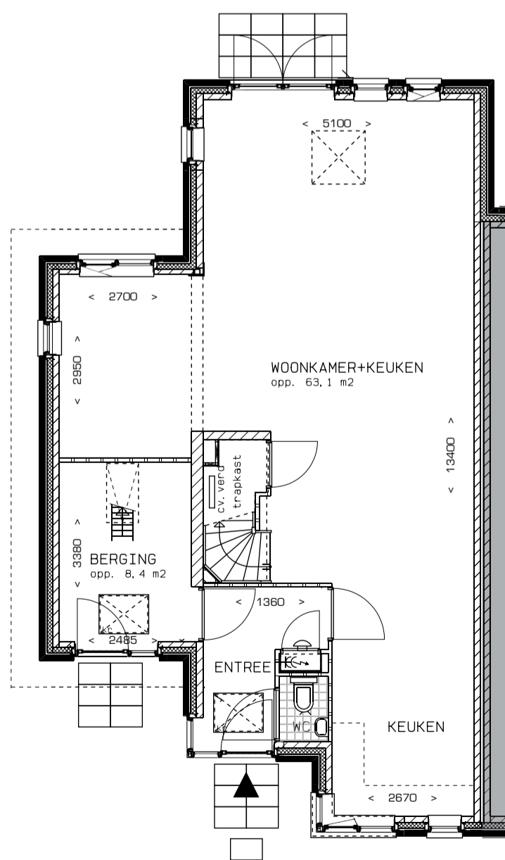
Begane grond • uitbouw 2400 mm achtergevel + lichtkoepel bouwnummers: 2, 6, 7, 10, 150 en 154 bouwnummers gespiegeld: 1, 3, 8, 9, 153 en 157 schaal 1 : 100
