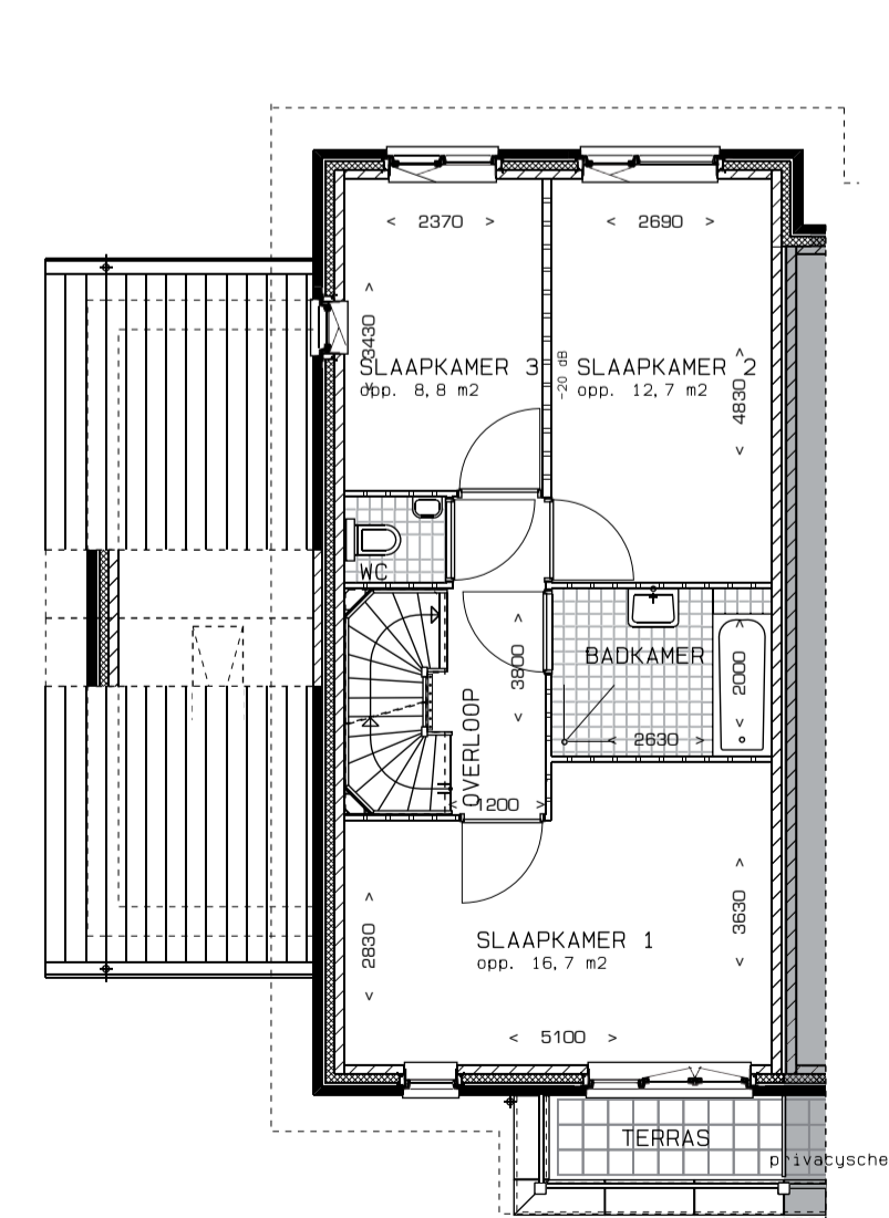
Eerste verdieping • uitbouw 900 mm bouwnummers: 2, 6, 7, 10, 150 en 154 bouwnummers gespiegeld: 1, 3, 8, 9, 153 en 157 schaal 1:100
