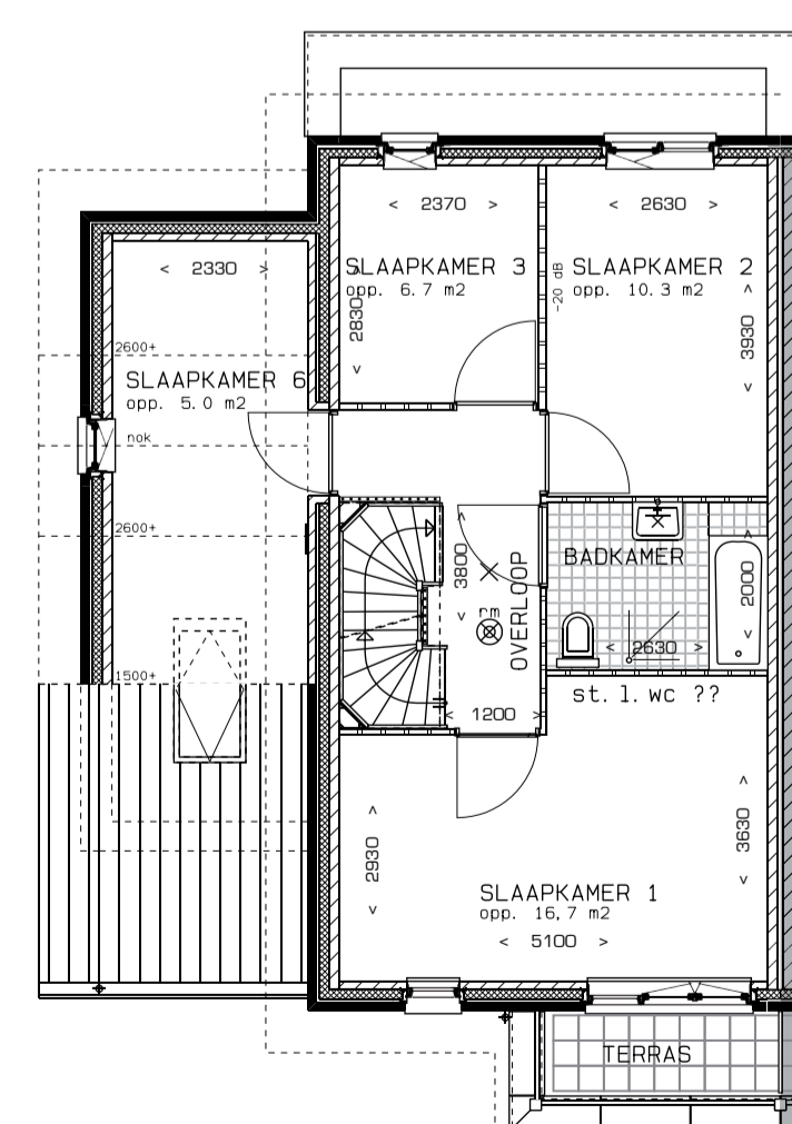
Eerste verdieping • dakraam extra slaapkamer 5 bouwnummers: 2, 6, 7, 10, 150 en 154 bouwnummers gespiegeld: 1, 3, 8, 9, 153 en 157 schaal 1 : 100
