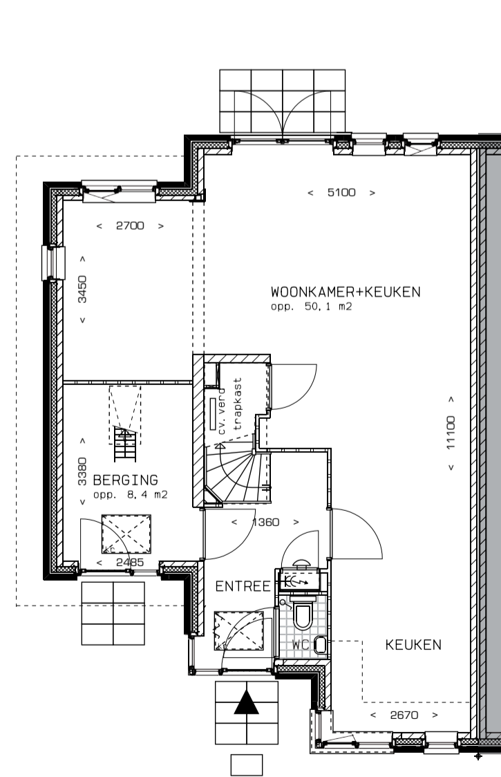
Begane grond • trap in entreehal bouwnummers: 2, 6, 7, 10, 150 en 154 bouwnummers gespiegeld: 1, 3, 8, 9, 153 en 157 schaal 1:100
