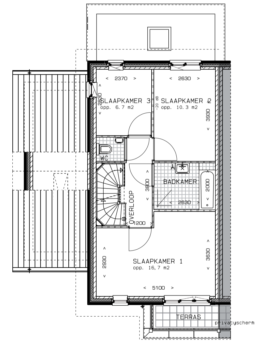
Eerste verdieping • dak uitbouw 2400 mm + lichtkoepel bouwnummers: 2, 6, 7, 10, 150 en 154 bouwnummers gespiegeld: 1, 3, 8, 9, 153 en 157 schaal 1:100
